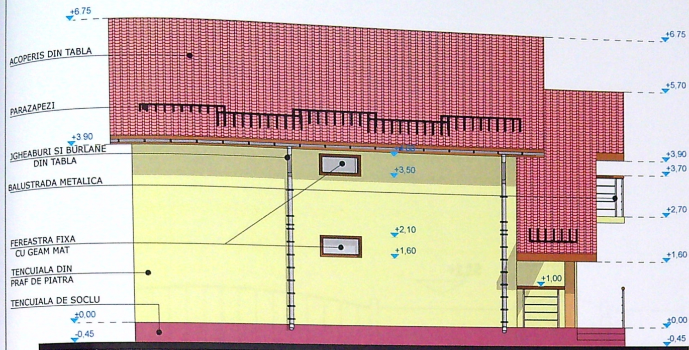
FATADA EST SCARA 1:100
